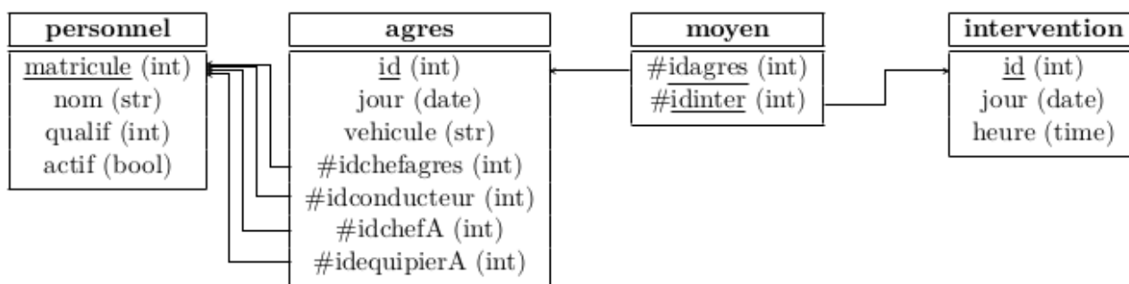
Figure 1. Schéma relationnel
